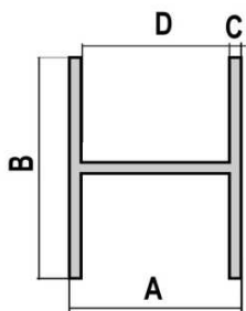
Profil H
