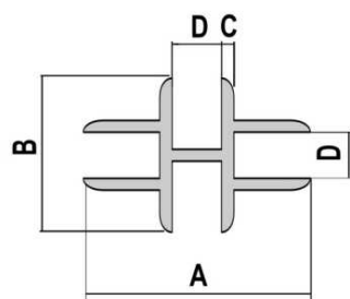
Profil křížový
